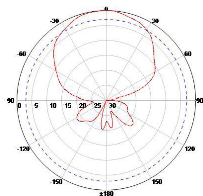
Вертикальная, 3 дБ
