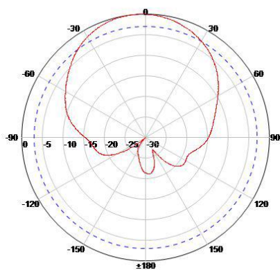
Горизонтальная, 3 дБ
