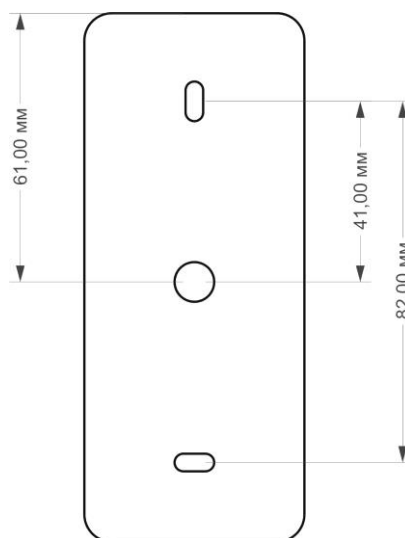
Монтажный чертёж
